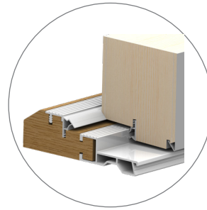
Tippanokka ohjaa veden pois ovilehdestä. Vesipelti on helppo kiinnittää kynnykseen.
