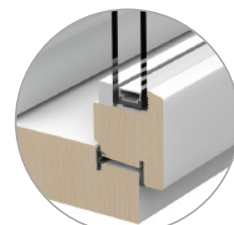
Suorareunainen sisäpuite
