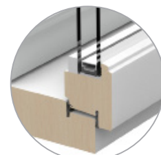
Koristekeilattu sisäpuite
